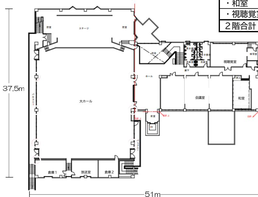
[2階]
